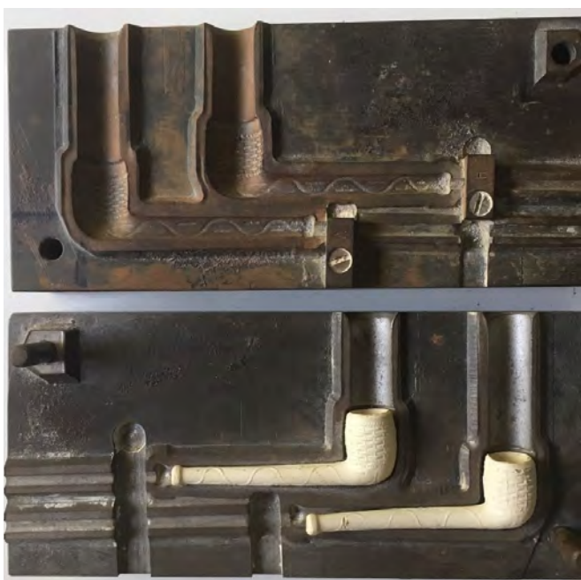
Afb. 25. Mal van de volautomatische machine. Foto en collectie auteur.
